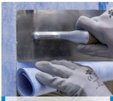
Przyklejanie drugiego arkusza membrany
